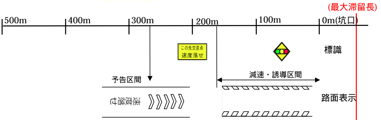
(a) シークエンスデザインの展開案と、交通安全施設の配置
